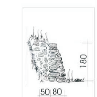
Sezione del muro ripristinato
