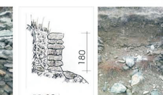
sezione del muro da ripristinare
